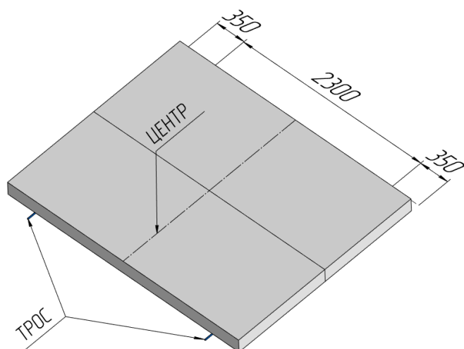
Рисунок 2 – Закладка тросов
