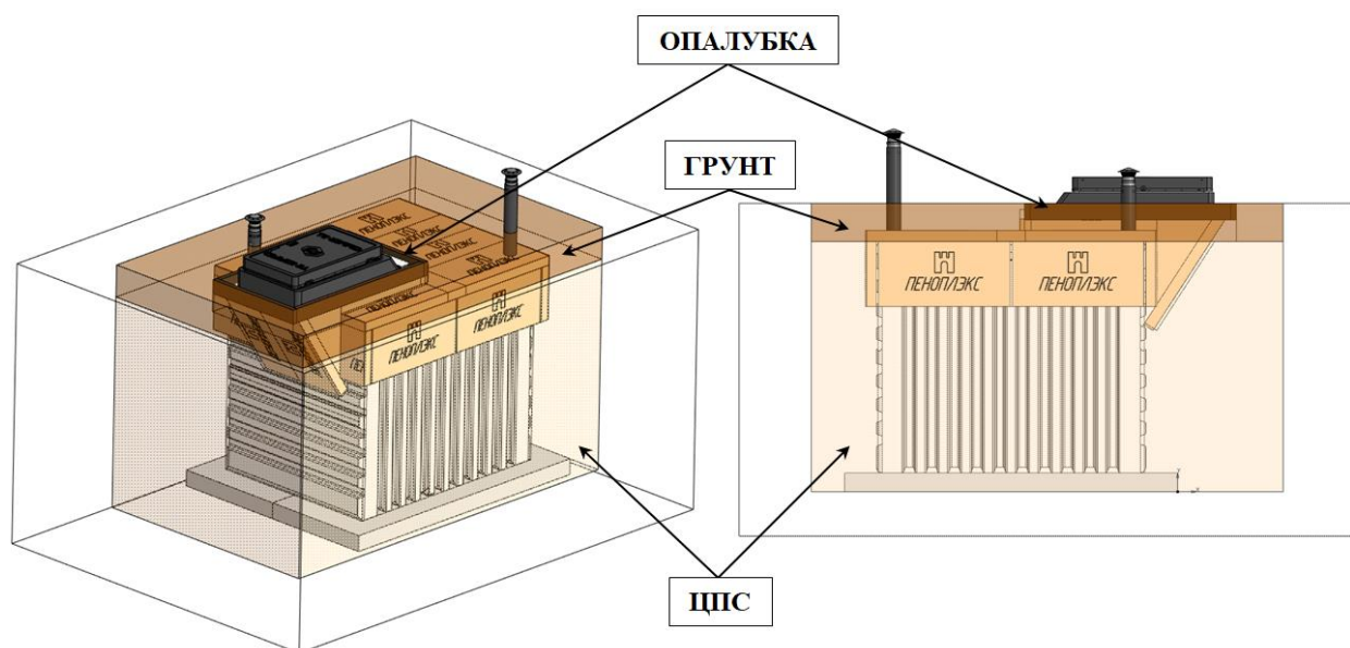
Рисунок 12 – Засыпка погреба
