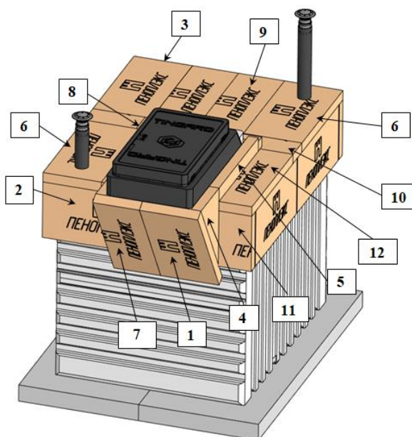
Рисунок 8 – Схема монтажа утеплителя
